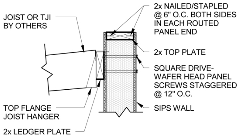
1 LEDGER DETAIL D29 1" = 1'-0"
